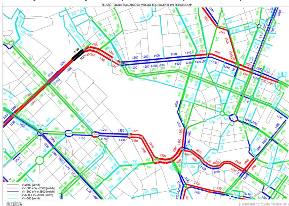
Figura 5-61 – Flussogramma del quadrante urbano di riferimento – Stato di fatto AM
