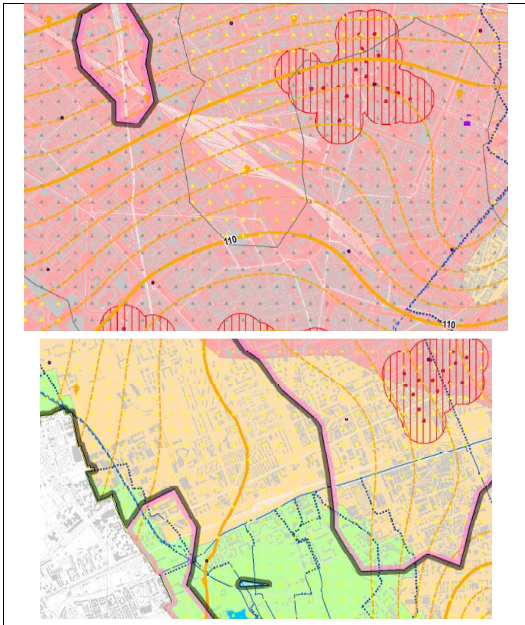
Figura 5-21 – Tavola G.03: Carta idrogeologica - Componente geologica, idrogeologica e sismica del PGT “Milano 2030”
