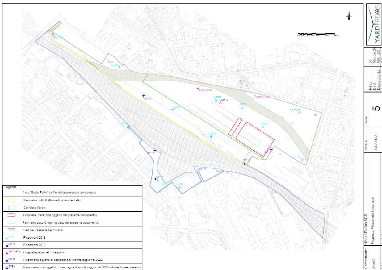
Figura 5-32 - Rete piezometrica – Esistente e di nuova installazione (PdC approvato con determina prot. N. 459452 del 06/09/2024)
