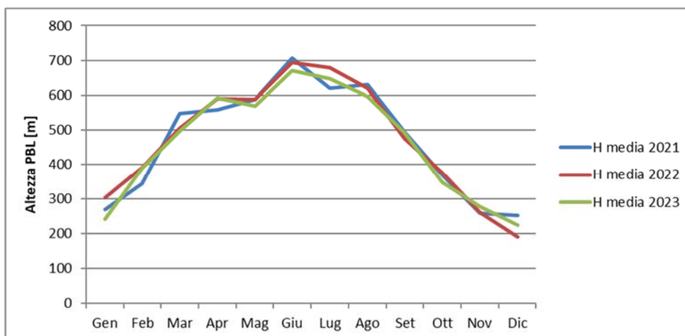
Figura 5-28 - Altezza strato di rimescolamento media mensile – Corsico Viale Italia
