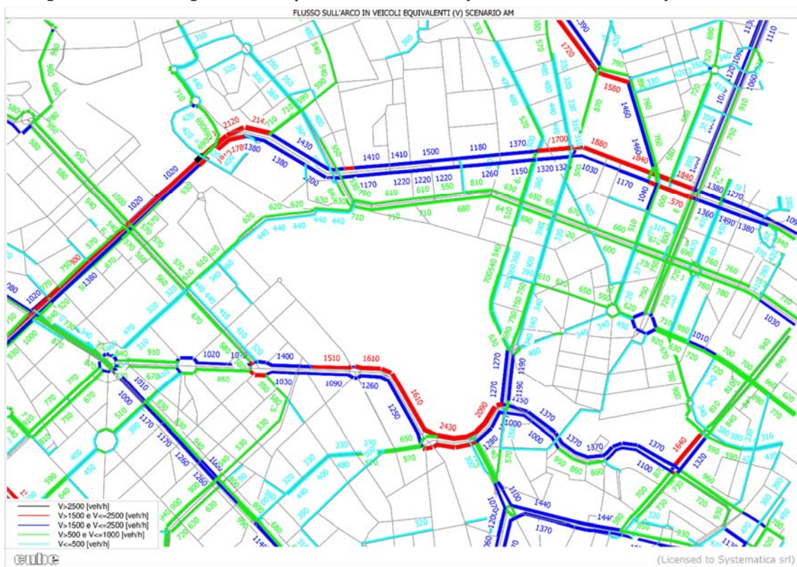
Figura 5-69 – Flussogramma nel quadrante urbano di riferimento – Scenario di riferimento AM
