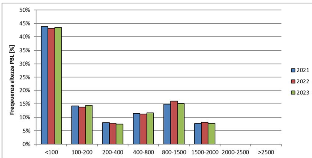
Figura 5-29 - Frequenza altezza strato di rimescolamento – Milano Brera
