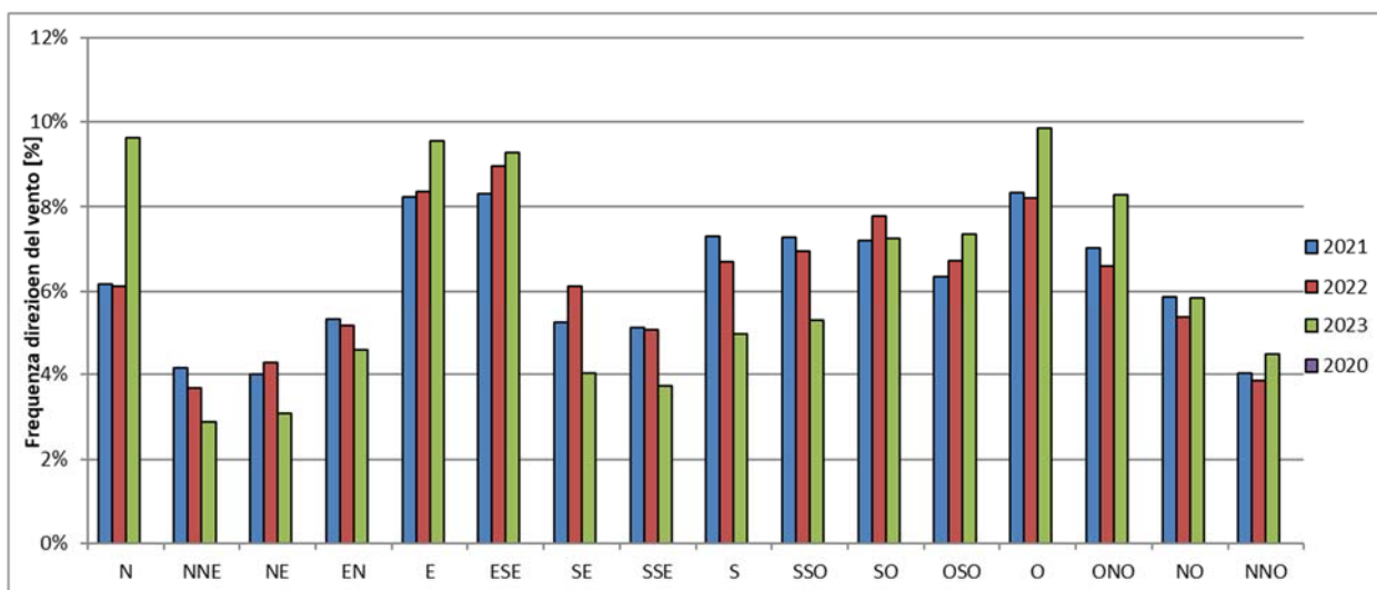
Figura 5-19 - Rosa dei venti (destinazione del vento) – Corsico Viale Italia
