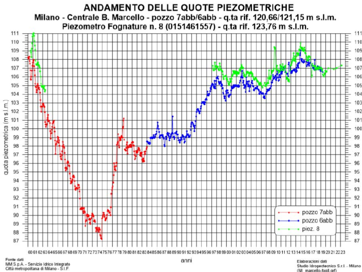
Figura 5-25 – Andamento delle quote piezometriche
