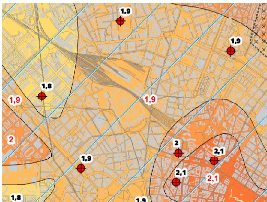
Figura 5-35 – Stralcio della Tavola G12: Carta dei fattori di amplificazione 0.5 - 1.5 e di confronto tra fa calcolati e da normativa - Componente geologica, idrogeologica e sismica del PGT "Milano 2030"
