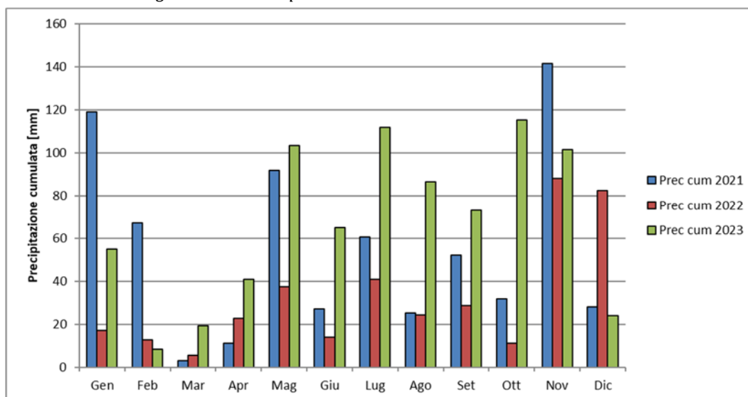
Figura 5-24 - Precipitazioni cumulate mensili – Milano Brera
