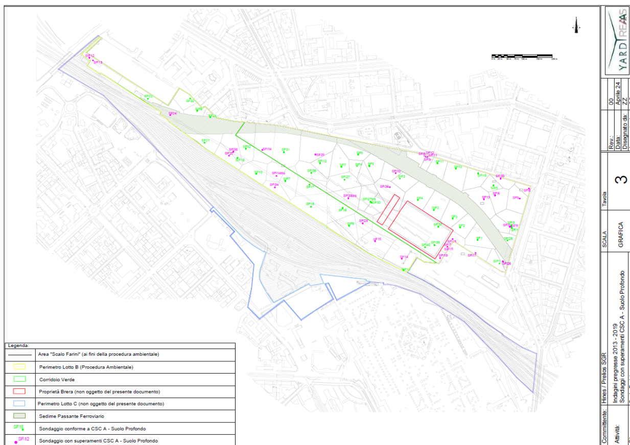
Figura 5-30 - Indagini eseguite e relativi superamenti riscontrati durante le caratterizzazioni passate (2013-2019)
