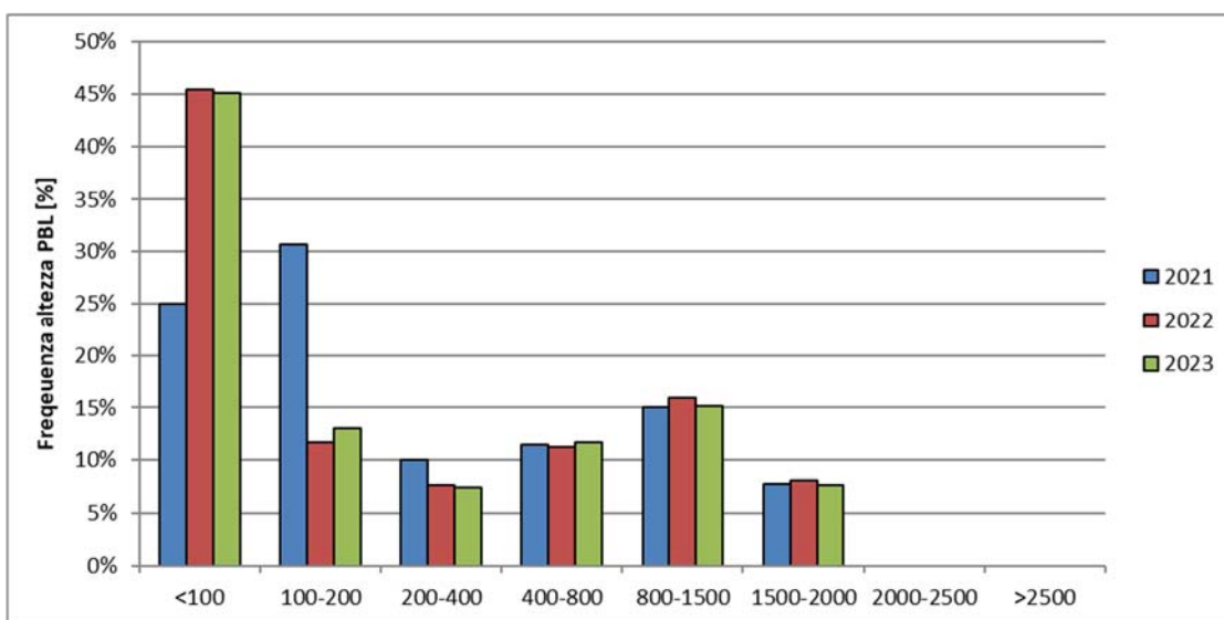
Figura 5-30 - Frequenza altezza strato di rimescolamento – Corsico Viale Italia
