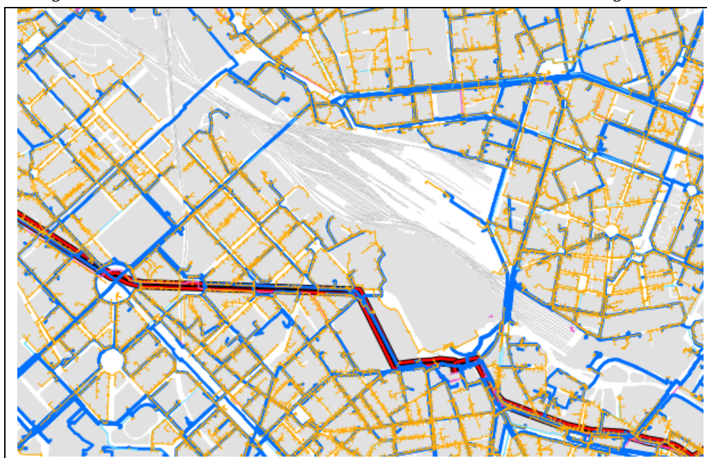
Figura 5-88 – Tavola T.01a del PUGSS: Sistema dei servizi a rete - Rete energia elettrica
