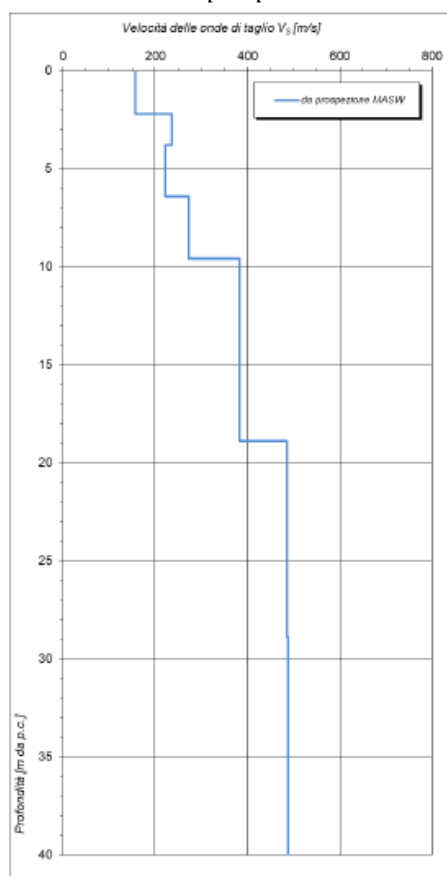
Figura 5-40 – Risultati prospezioni sismiche MASW
