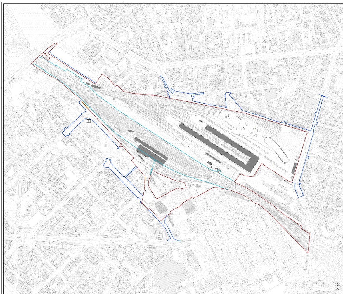
Figura 1-3 – Inquadramento delle aree di intervento
