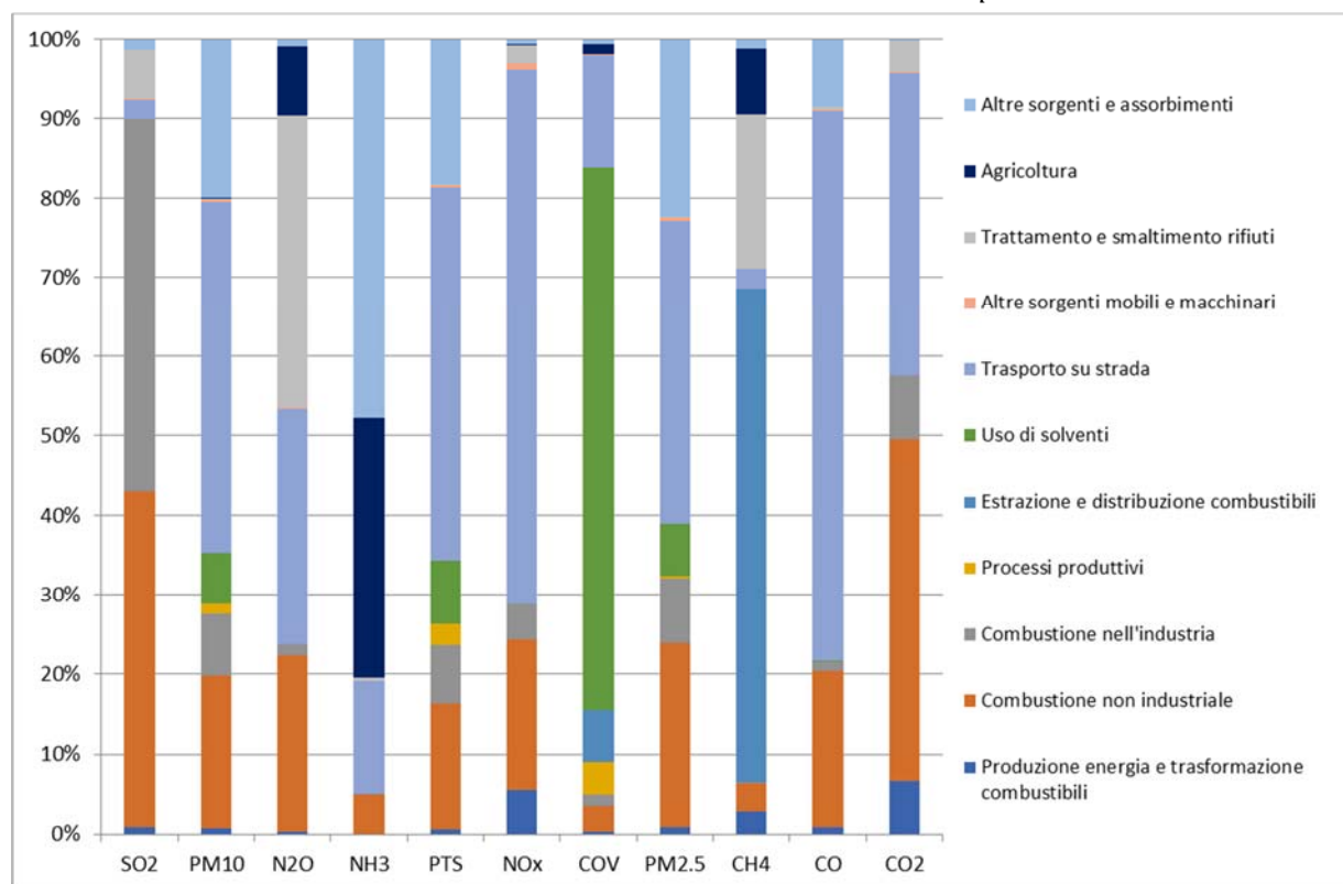
Figura 5-11 - Contributi percentuali alle emissioni per settore nel comune di Milano - INEMAR ARPA Lombardia - Emissioni in Lombardia nel 2021 - versione in revisione pubblica
