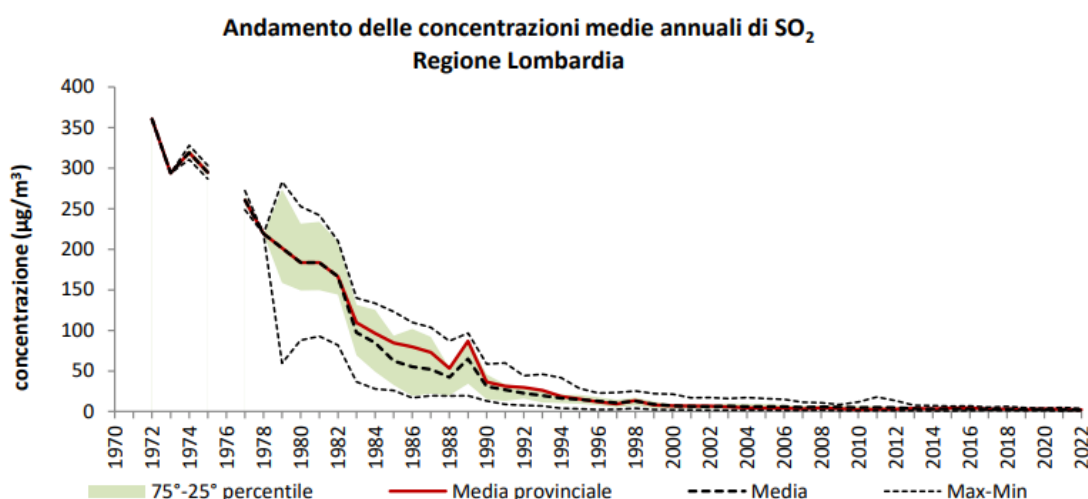
Figura 5-3 - Andamento delle concentrazioni medie annuali di SO 2 – Rapporto annuale sulla qualità dell'aria: anno 2022.
