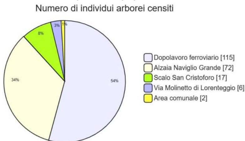
Figura 5-48 – Numero di individui arborei censiti nel perimetro di intervento, incluse le aree esterne al perimetro di proprietà
