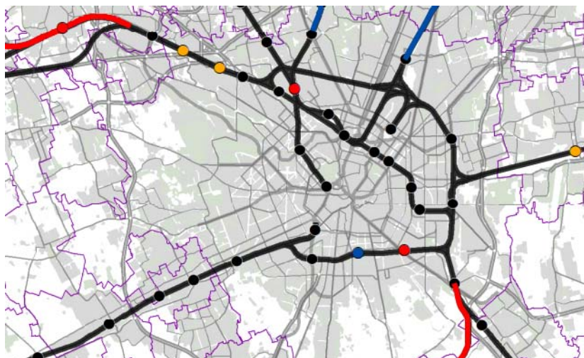
Figura 4-51 – Schema di riassetto della rete ferroviaria
