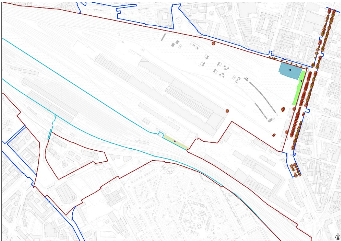
Figura 5-44 – Rilievo del verde esistente scalo Farini - 2
