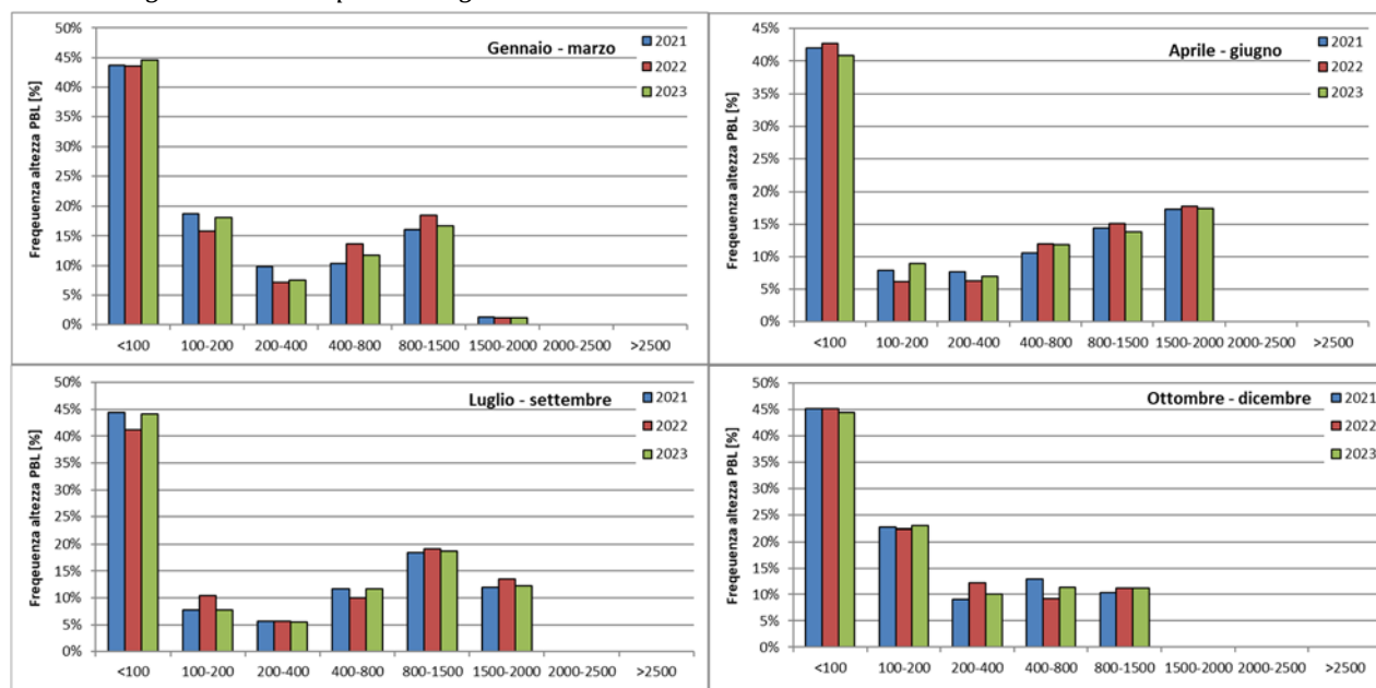
Figura 5-31 - Frequenza stagionale dell'altezza dello strato di rimescolamento – Milano Brera
