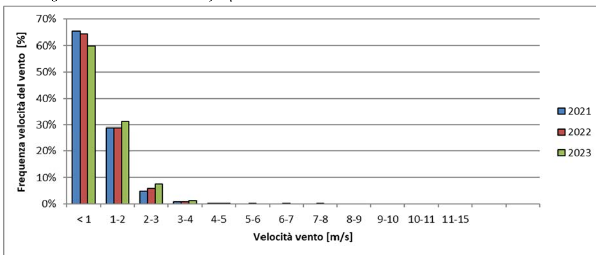
Figura 5-21 - Distribuzione di frequenza delle classi di velocità del vento – Corsico Viale Italia
