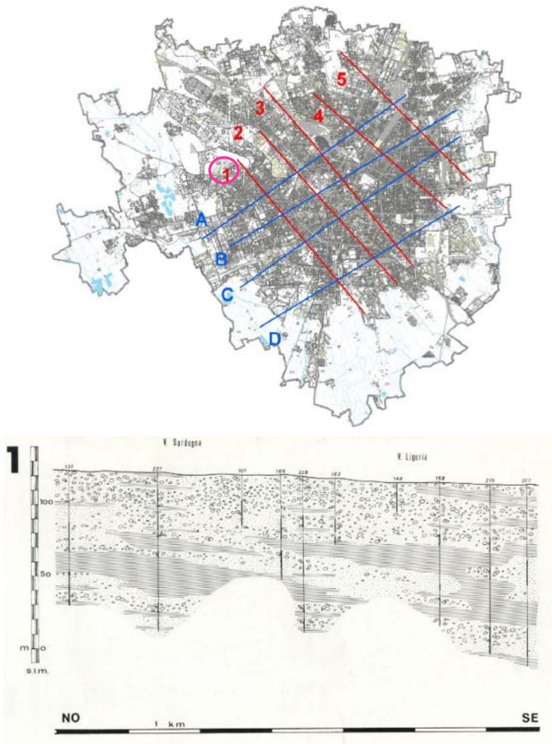
Figura 5-20 – Sezioni idrologiche pubblicate dalla Provincia di Milano rappresentative dell'acquifero milanese - Relazione illustrativa e norme geologiche di piano – PGT "Milano 2030"
