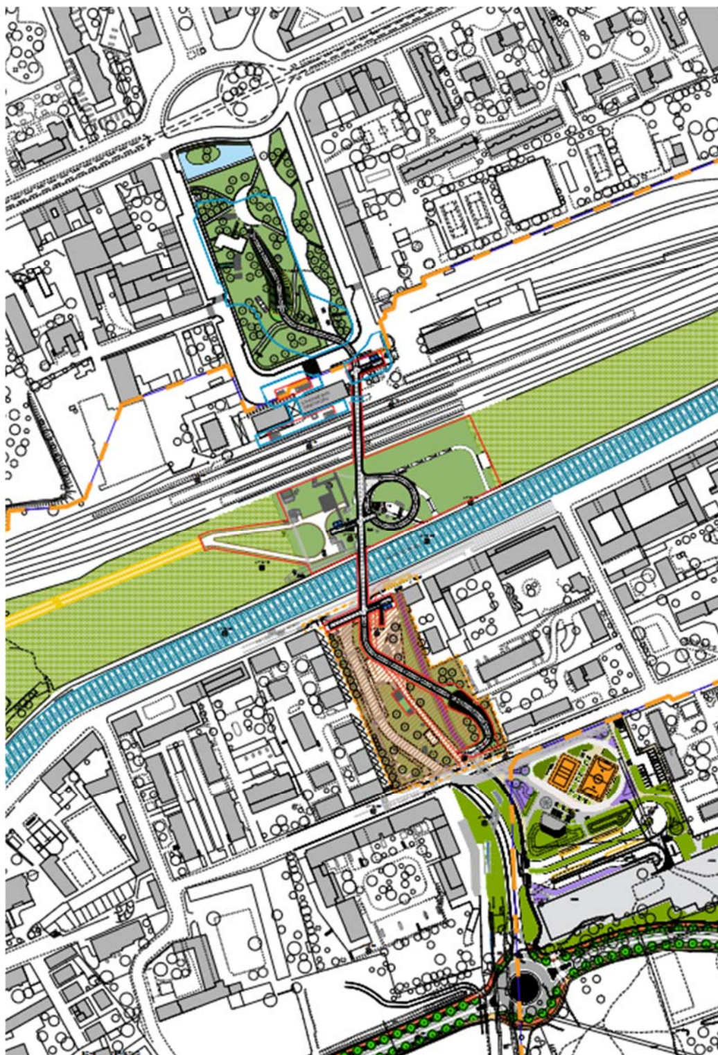
Figura 5-81 – Passerella ciclo-pedonale Stazione San Cristoforo – progetto esecutivo – fonte: Comune di Milano / M4 SPA
