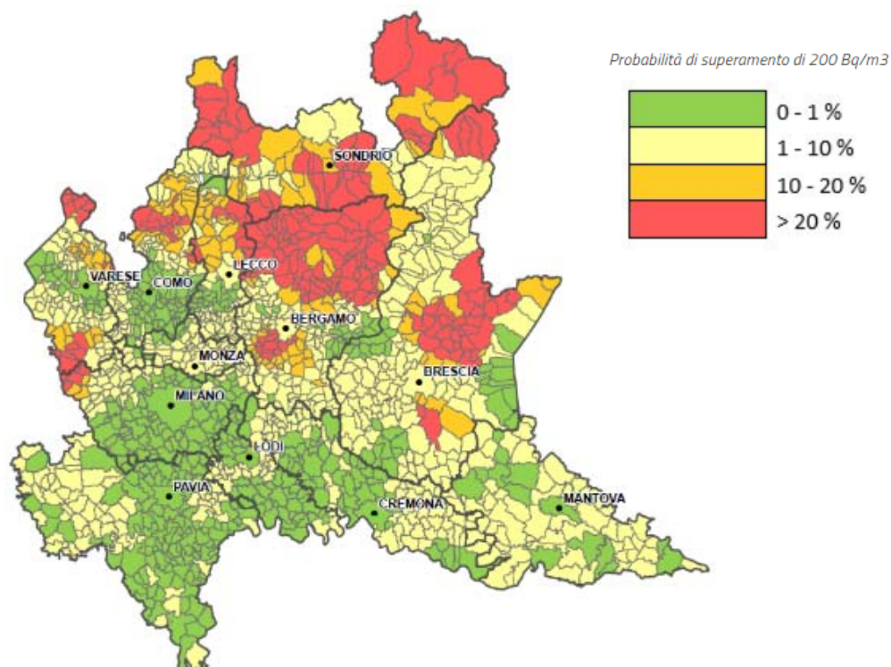
Figura 5-89 – Mappa della probabilità che una generica abitazione a piano terra abbia una concentrazione di radon superiore a un livello ritenuto significativo (200 Bq/m 3 )
