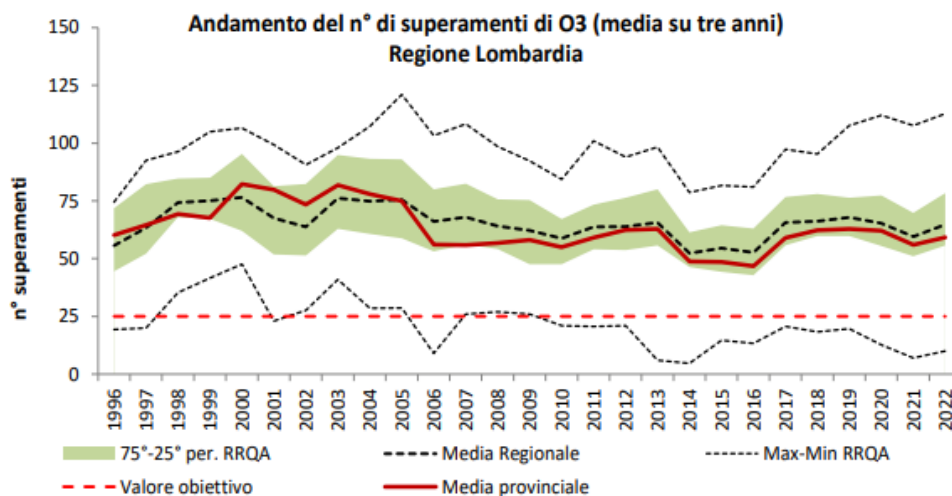
Figura 5-6 - Andamento del numero di superamenti annuali di O_3 – Rapporto annuale sulla qualità dell'aria: anno 2022.
