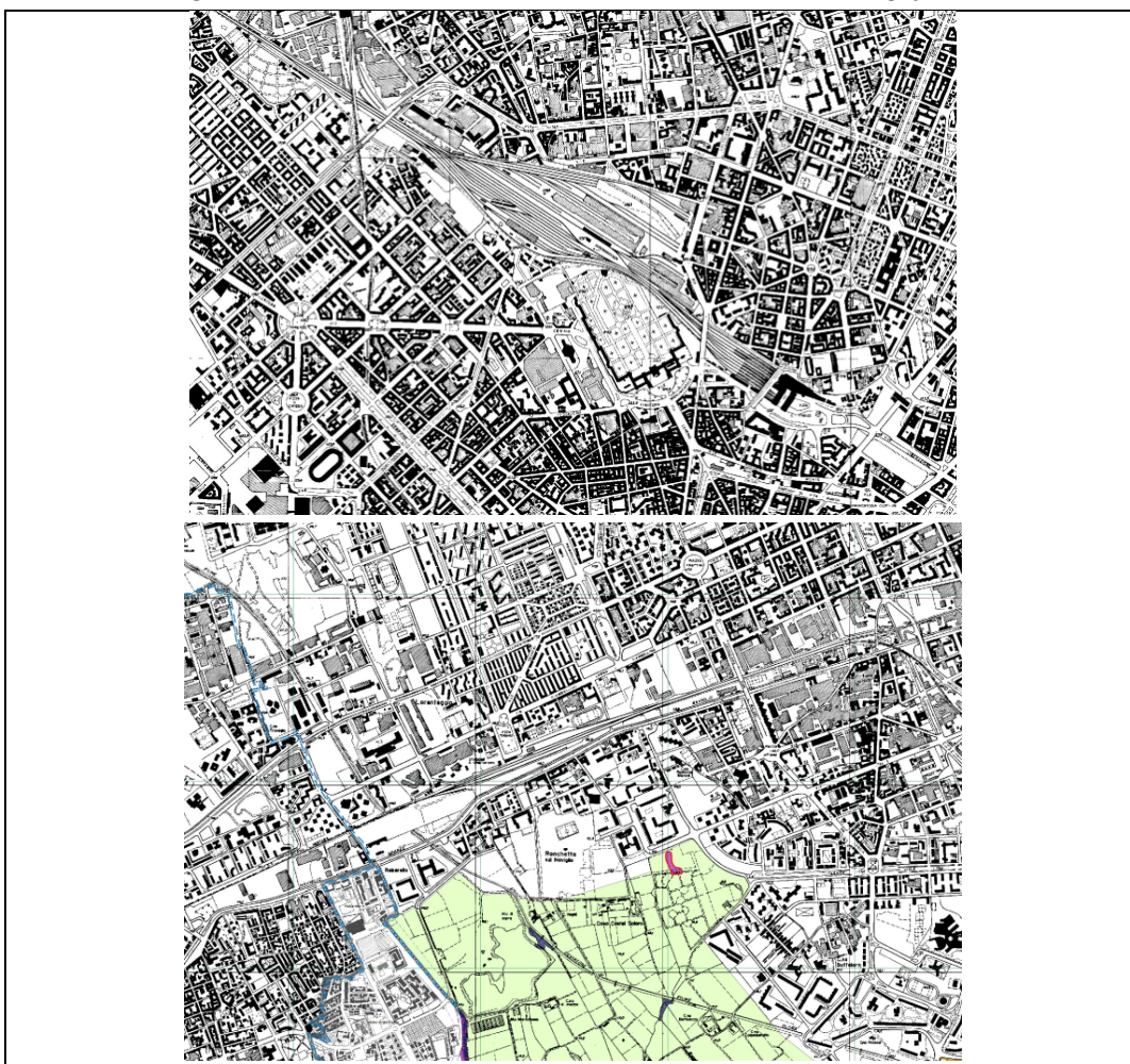
Figura 4-57 – Stralcio della Tavola 1: Carta dei boschi e dei tipi forestali
