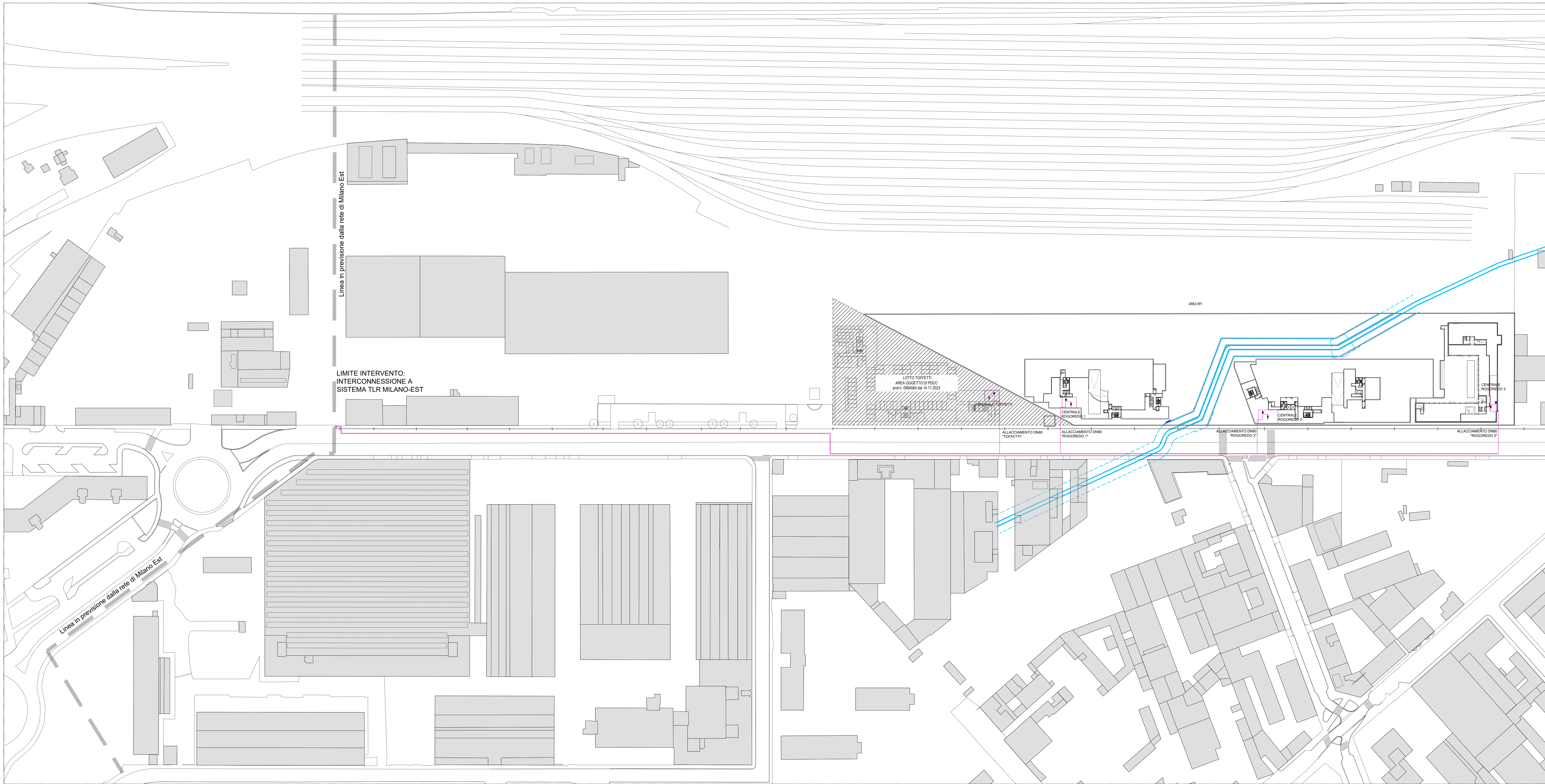
PLANIMETRIA STATO DI PROGETTO | SOTTOSERVIZI | TELERISCALDAMENTO SCALA 1:1000
