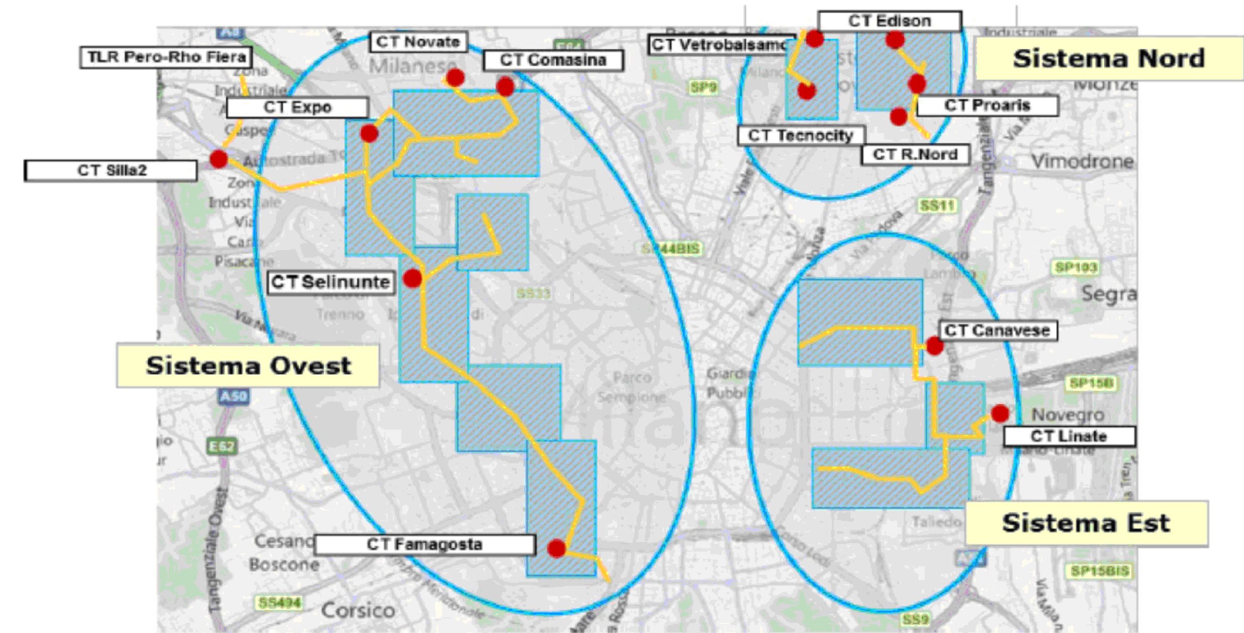
Sviluppo della rete di TLR pianificato dal Gruppo A2A Fonte: "Il Teleriscaldamento per l'area metropolitana di Milano: un grande progetto a rilevanza nazionale". A2A, Comune di Milano
